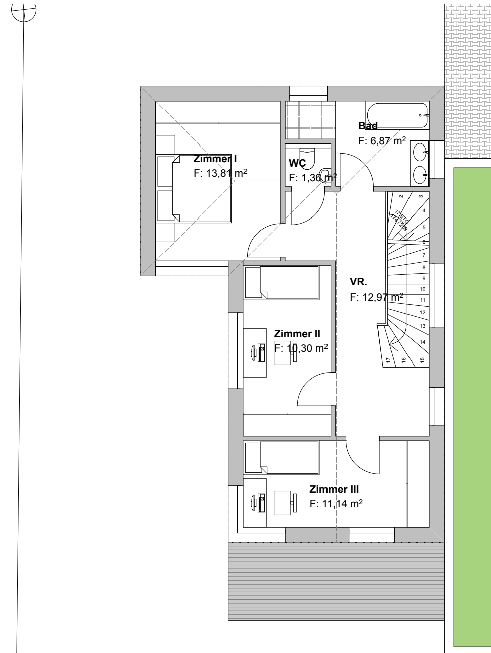
Haus 1 OG
